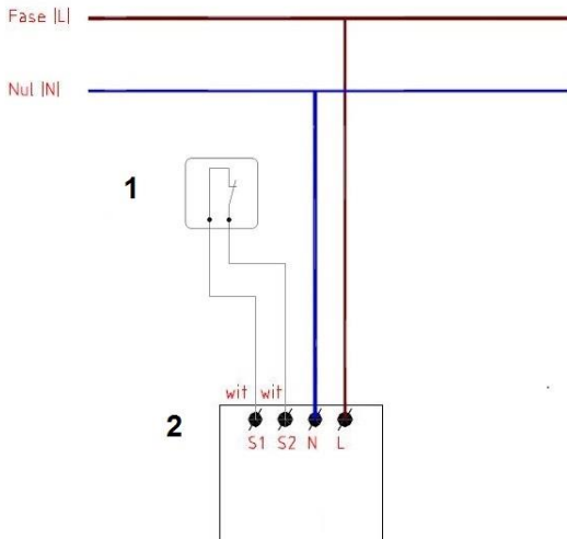
Afbeelding 2 – Aansluitschema voor één glasbreuksensor
