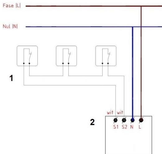
Afbeelding 3 – Aansluitschema voor meerdere glasbreukmelders
