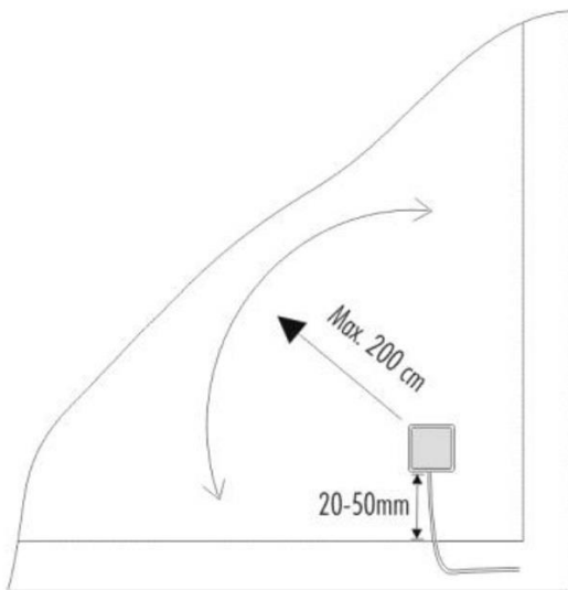
Afbeelding 1 – Montageplaats van de glasbreuksensor
