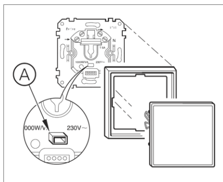
Afbeelding 2: Monteren van het bedieningsvlak
