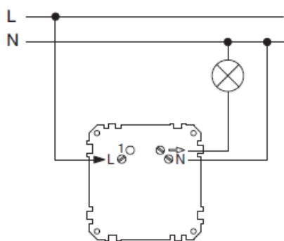
Afbeelding 1: Aansluiten van de sokkel
