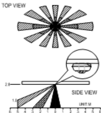
Image 10. Montage au plafond
