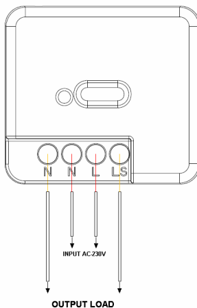
Figura 2. Esquema técnico
