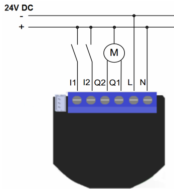
Afbeelding 1: Aansluitschema 24VDC motor
