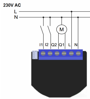
Afbeelding 2: Aansluitschema 230V AC motor
